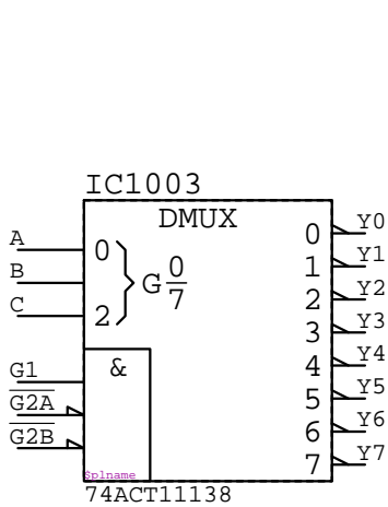
74ACT11138
