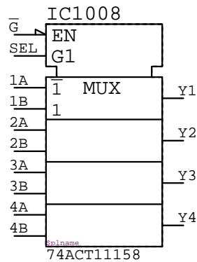
74ACT11158
