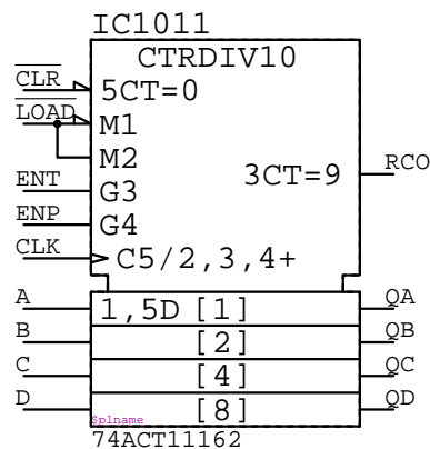
74ACT11162
