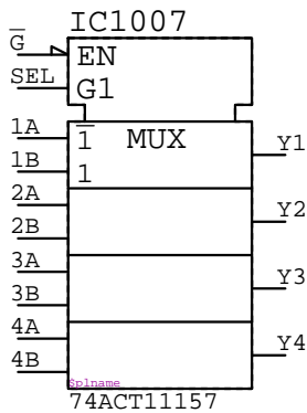
74ACT11157
