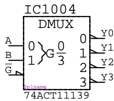
74ACT11139
