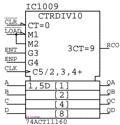
74ACT11160
