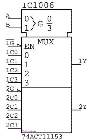
74ACT11153
